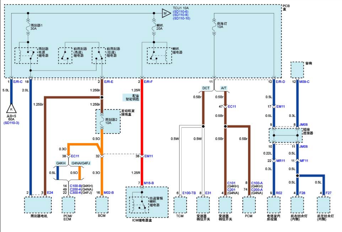
电源分布(4)
